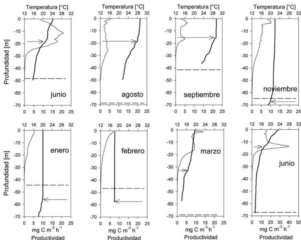
Figura 5. Perfiles verticales de temperatura (línea gruesa) y de productividad primaria (línea delgada). La flecha indica la profundidad de la capa de mezcla y el sentido hacia la derecha calentamiento, y hacia la izquierda enfriamiento. La línea quebrada indica la profundidad crítica.
