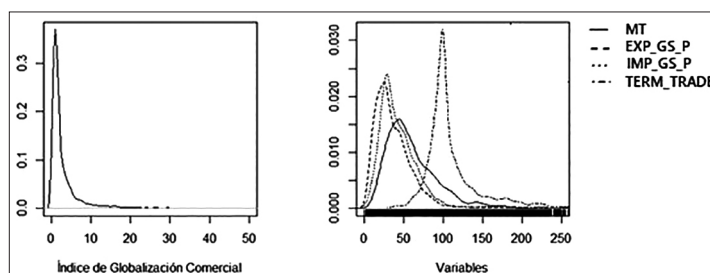
Figura 1. Distribución del Índice de Globalización Comercial.
