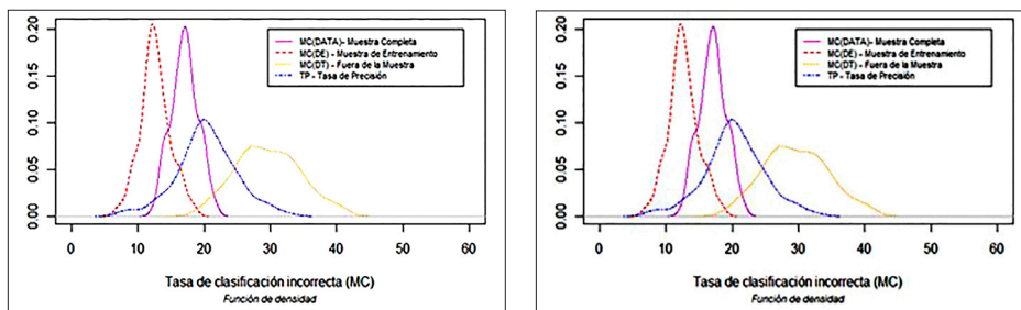
Figura 2. Distribución de las medidas de ajuste de los modelos.
