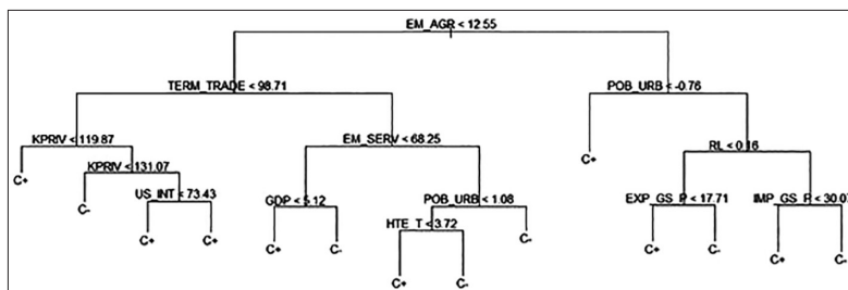
Figura 3. Representación Gráfica del Árbol Clasificador.
