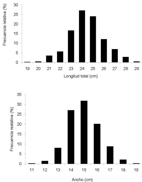
Figura 3. Frecuencias relativas de peso total (a) y del músculo aductor (b) de Atrina oldroydii .
