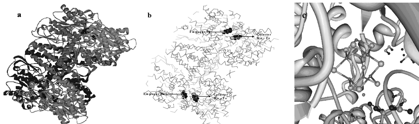
Figura 2. Comparación de vistas de la proteína Mo-Fe en la proteína obtenida de Klebsiella pneumoniae (Mayer, 1999). (a) vista de cadenas como sustituyentes; (b) vista con los cúmulos metálicos expuestos, y (c) vista del cofactor en el entorno proteínico.
