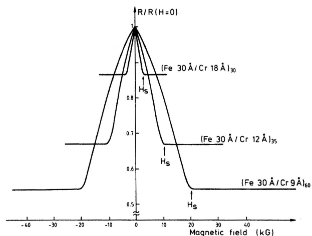
Figura 1. Medida original de Fert y colaboradores (Baibich et al. , 1988; Binasch et al. , 1989) en donde se observa el abatimiento de la resistencia eléctrica al aumentar el campo magnético.
