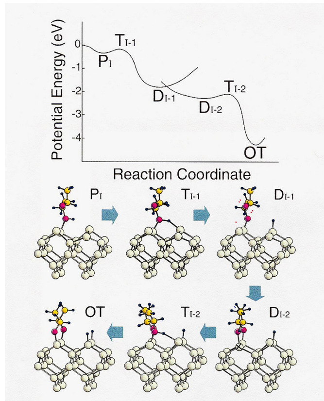
Figura 3. Perfil de energía de la reacción de fisisorción de 2,3-butanediol en una superficie de Si (001) (Lee y Cho, 2007).
