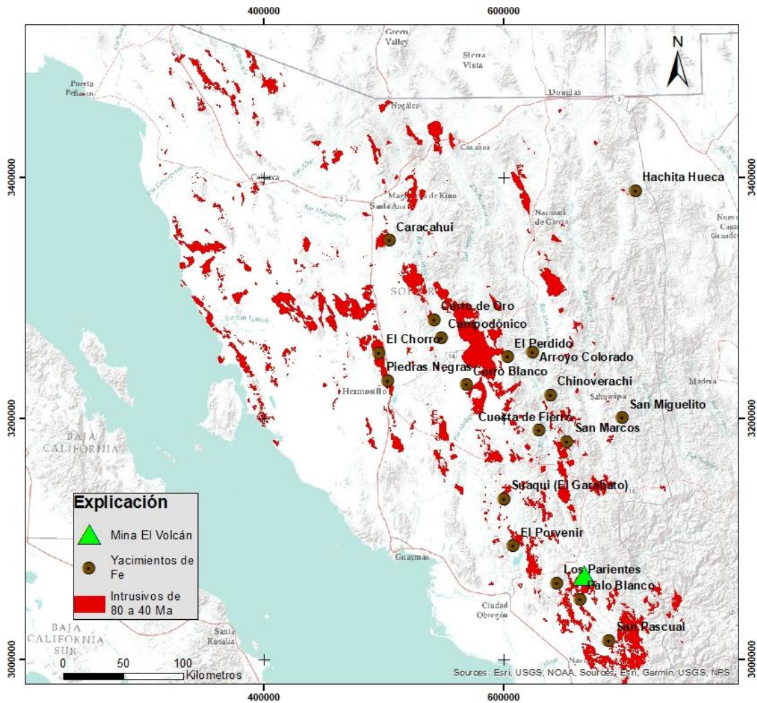
Figura 1. Distribución de los yacimientos de Fe en Sonora.
