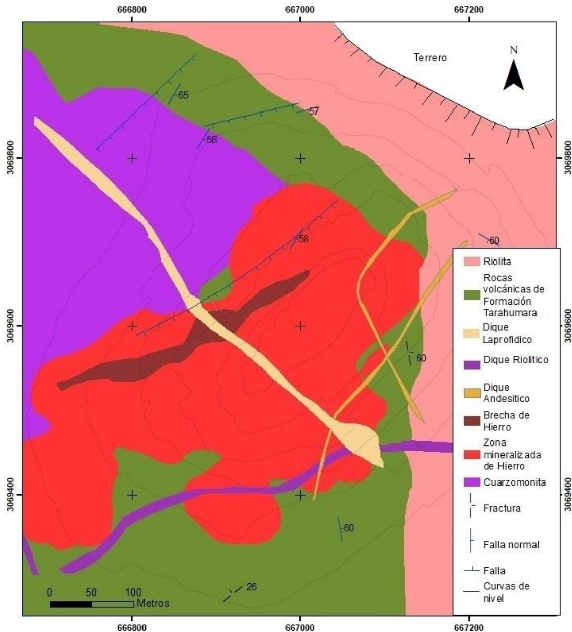
Figura 2. Geología del depósito El Volcán.
