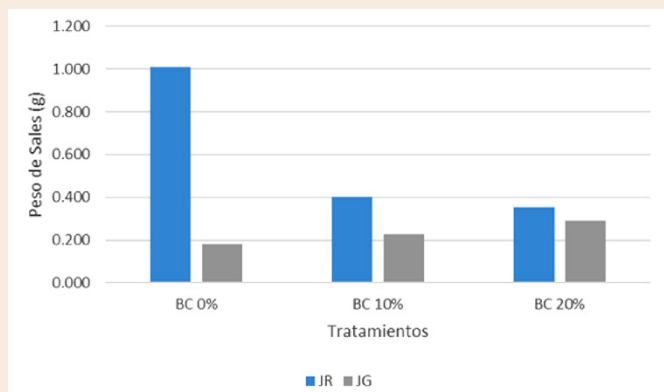
Figura 4. Resultados de la producción de sales eflorescentes por cada 25 ml de efluente, para las columnas con mezclas de Jales ricos en óxidos (JR) y jales ricos en sulfuro (JG) con bone char (BC).
