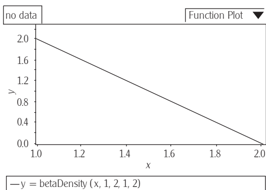
Figura 11 Distribuciones muestrales
