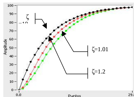
Fig. 6. Respuestas sobreamortiguadas.
