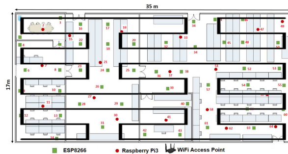
Fig. 9. Distribución de UMC en una planta convencional utilizando la curva fractal de Peano
