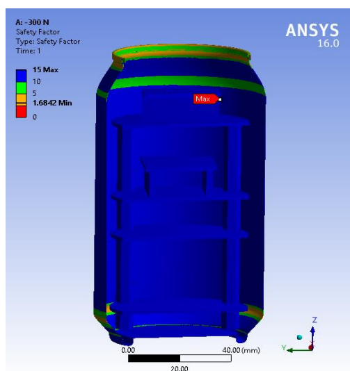
Fig. 9. Factor de seguridad de estructura CanSat
