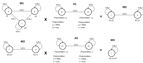
Fig. 7. Update of M1 with A1 and A2
