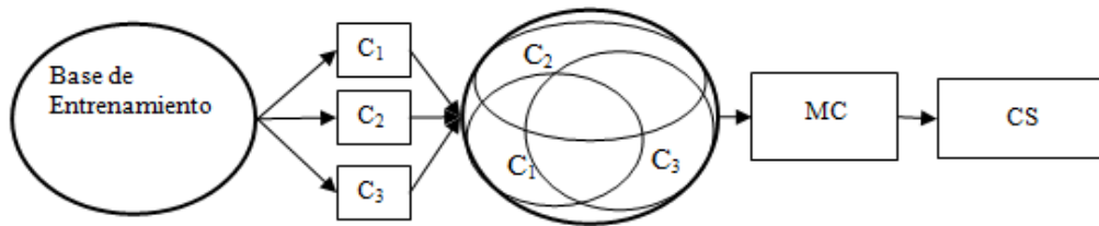
Fig. 1 Ejemplo de un modelo multclasificador basado en conjuntos de instancias bien clasificadas con tres clasificadores de bases
