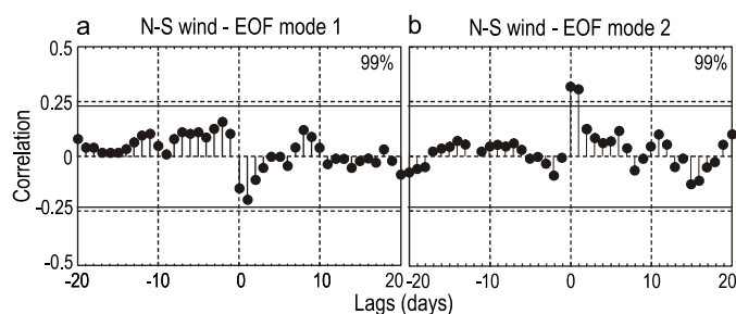
Figura 10. Correlación cruzada entre el estrés del viento norte-sur y el modo 1 (a) y entre el estrés del viento y el modo 2 (b) de la variabilidad de la temperatura. El nivel de confianza utilizado es 99%, sólo la correlación entre el estrés del viento y el segundo modo de FEO muestra valores significativos.
