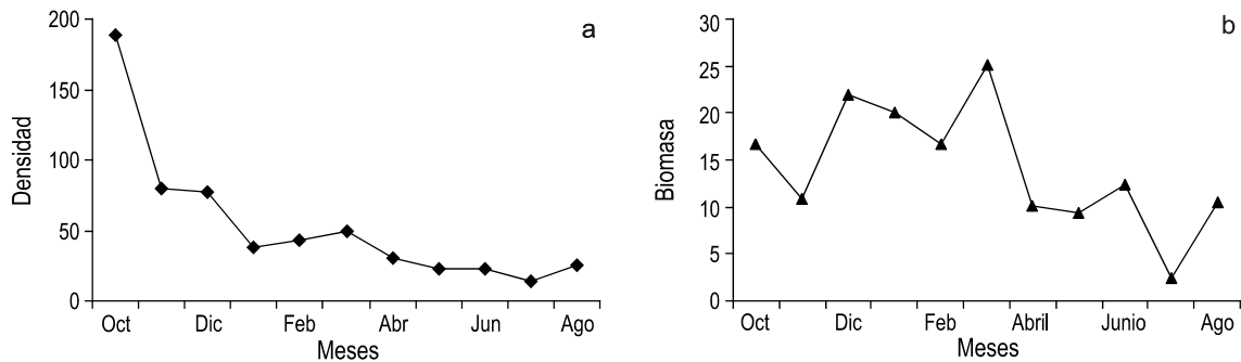
Figura 4. Variación de la densidad poblacional (ind m^{-2} ) y biomasa poblacional mensual (gPs m^{-2} ) de Tivela mactroides de Playa Caicara. Figure 4. Density (ind m^{-2} ) and biomass (gDW m^{-2} ) of Tivela mactroides from Caicara Beach.
