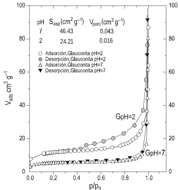
Figura 7. Análisis BET de las variaciones de superficie específica y porosidad. La disminución de S_{esp} y V_{poro} durante el ataque ácido está probablemente conectada con el proceso de disolución selectiva en los bordes de grano y la generación de componente amorfo.
