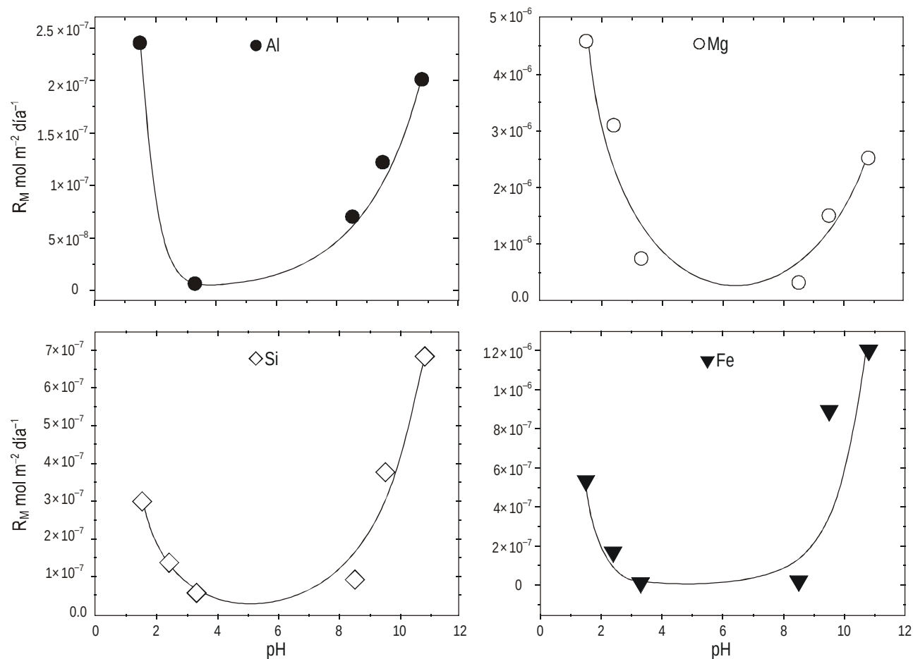
Figura 2. Variación de la constante de velocidad de disolución, R_M ( M = \text{Al, Mg, Si, Fe} ), en función del pH. R_M es el valor estacionario obtenido al final de cada experimento normalizado a su estequiometría en la fórmula de la glauconita. Las líneas representan el ajuste de los puntos experimentales a la expresión 5. Figure 2. Variation of the dissolution rate constant, R_M ( M = \text{Al, Mg, Si, Fe} ), relative to pH; R_M is the stationary value obtained at the end of each experiment normalized to its stoichiometry in the glauconite formula. The lines represent the fit of the experimental points to equation 5.
