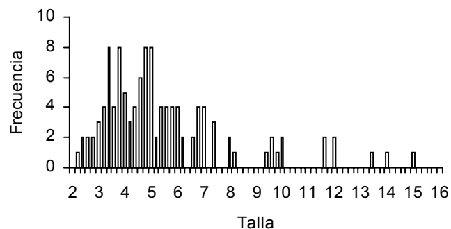
Figura 1. Estructura de tallas de la población de Lithothamnion muelleri de Punta Galeras, Golfo de California (México)
