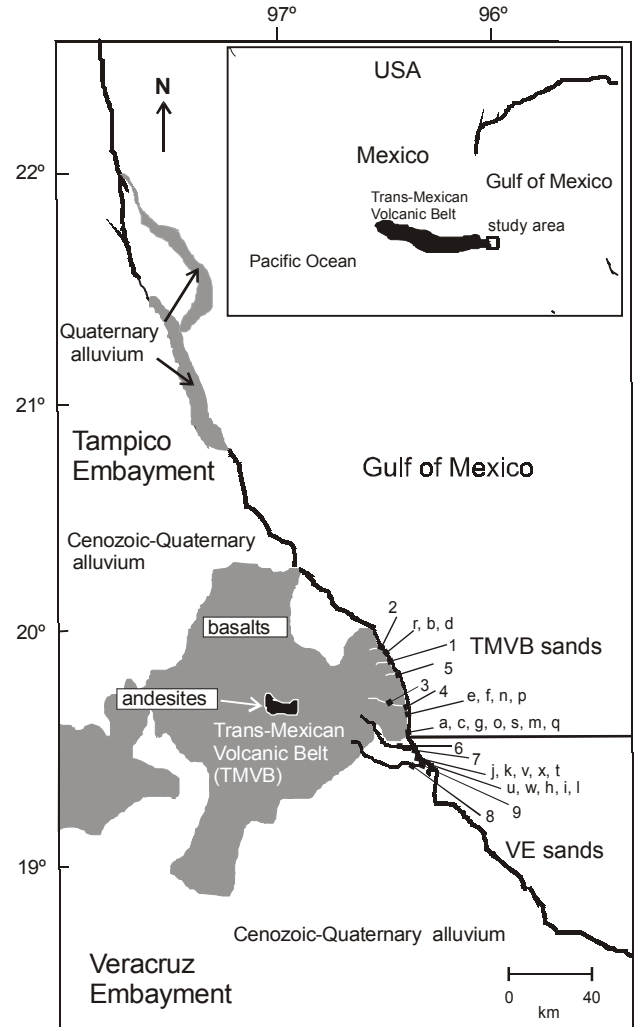
Figure 1. Geology and sampling sites of the study area. Figura 1. Geología del área de estudio y ubicación de los sitios de muestreo
