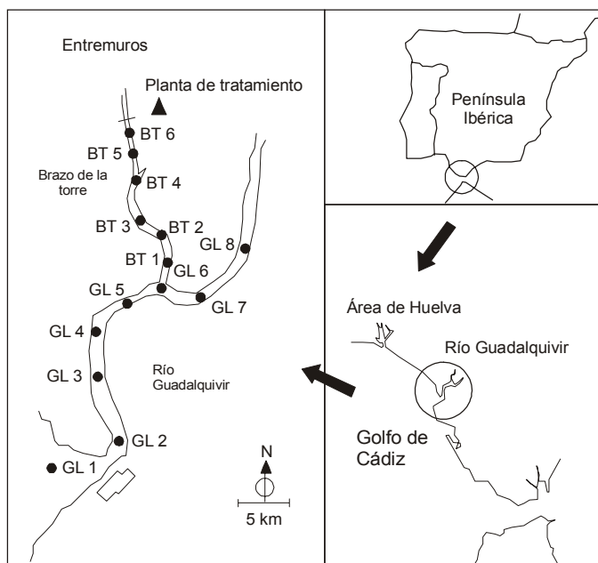
Figura 1. Localización geográfica de los ríos Guadalquivir y Guadamar (incluyendo el Brazo de la Torre) en la que se reseñan las distintas estaciones de muestreo.
