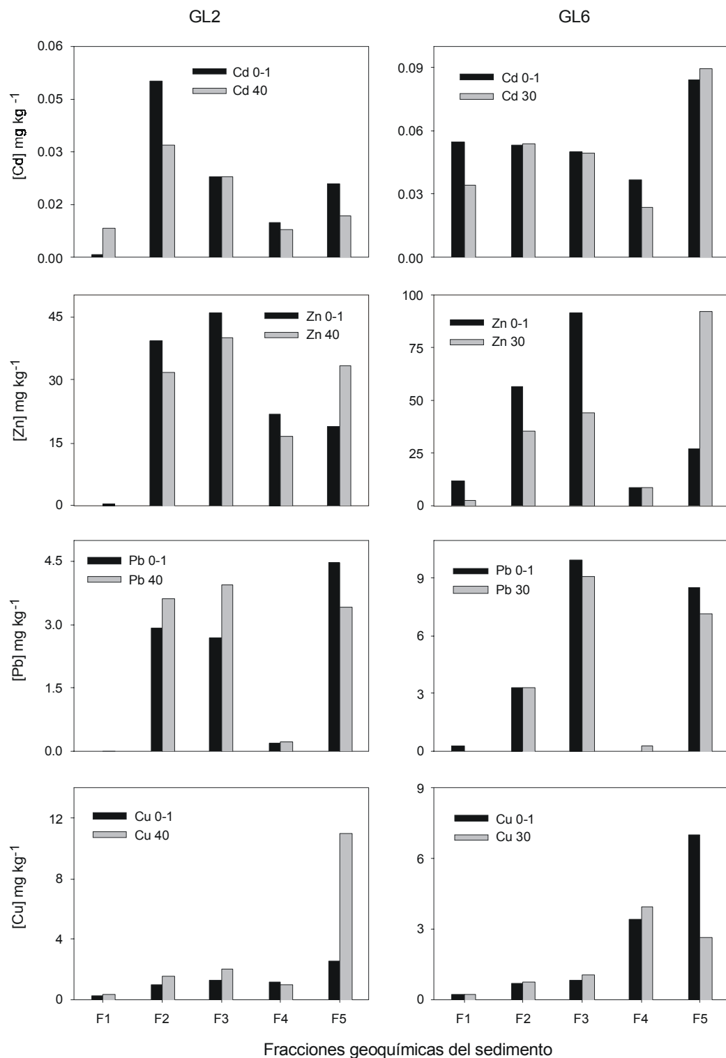
Figura 4. Concentración de metales pesados Cd, Zn, Pb y Cu (mg kg -1 ) asociada a las diferentes fracciones geoquímicas (F1–F5) de los sedimentos superficiales y profundos de las estaciones GL2 y GL6 localizadas en el estuario del Guadalquivir.
