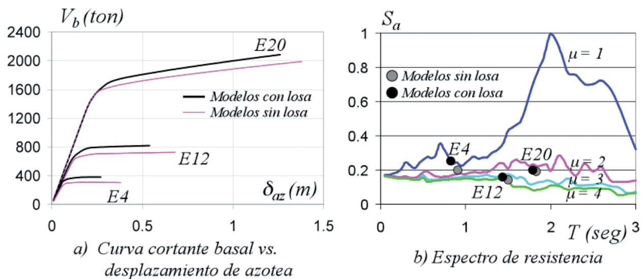
Fig. 5. Efecto de la losa en las propiedades estructurales de los edificios.
