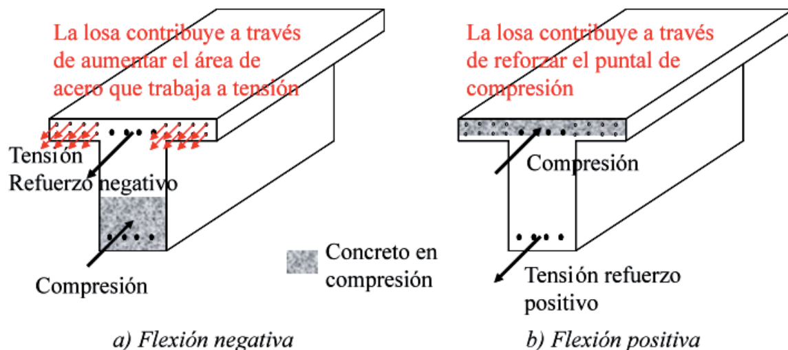
Fig. 1. Contribución de la losa a las características mecánicas de las vigas, flexión.
