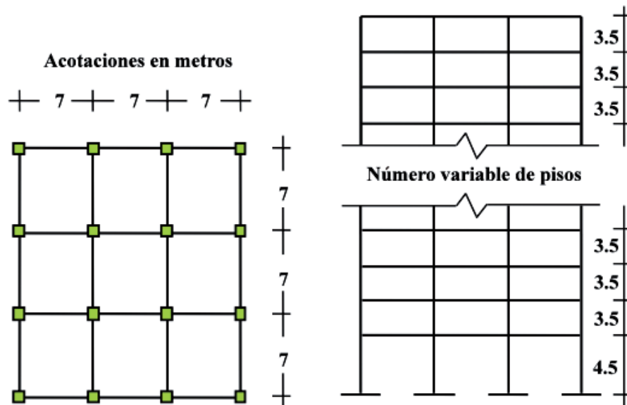
Fig. 2. Configuración estructural de los edificios considerados.
