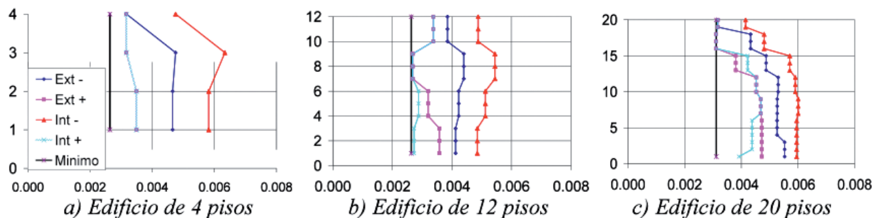
Fig. 3. Cuantías de acero en las vigas de los edificios.
