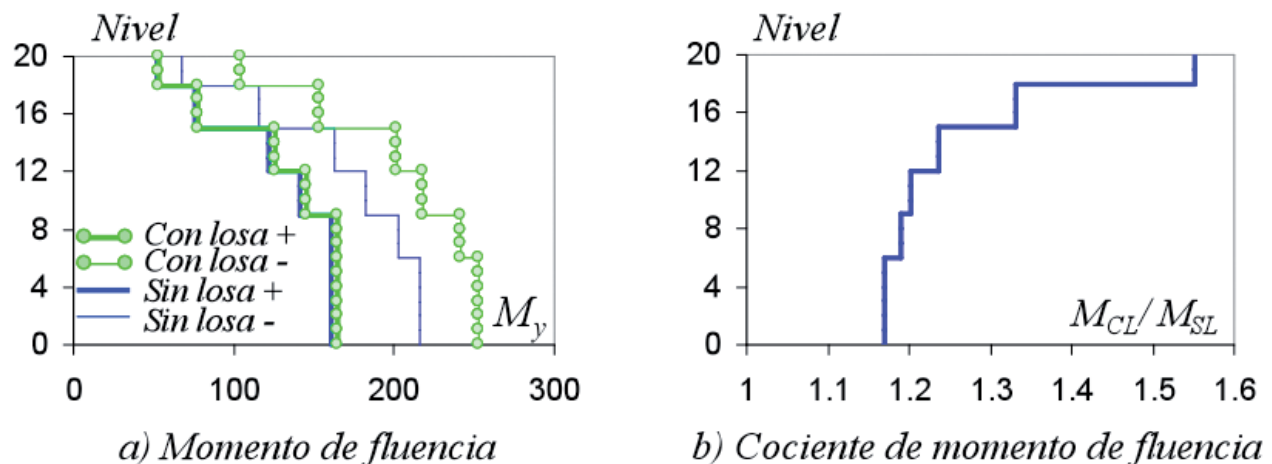
Fig. 7. Efecto de la losa en el momento de fluencia de las vigas de los marcos internos del edificio de veinte pisos.
