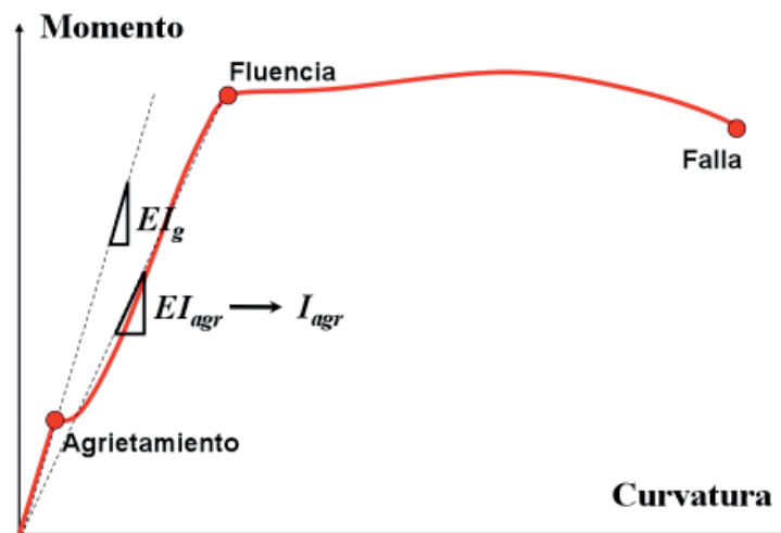
Fig. 4. Definición de momento de inercia agrietado para una sección transversal de concreto reforzado.
