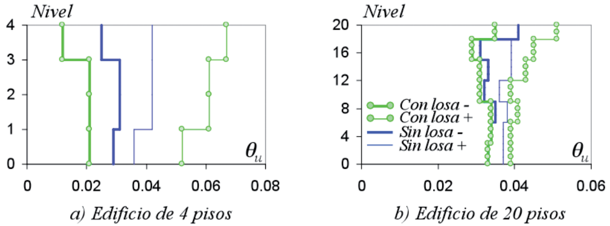
Fig. 8. Efecto de la losa en la capacidad de rotación última de las vigas de los marcos internos de los edificios de cuatro y veinte pisos.
