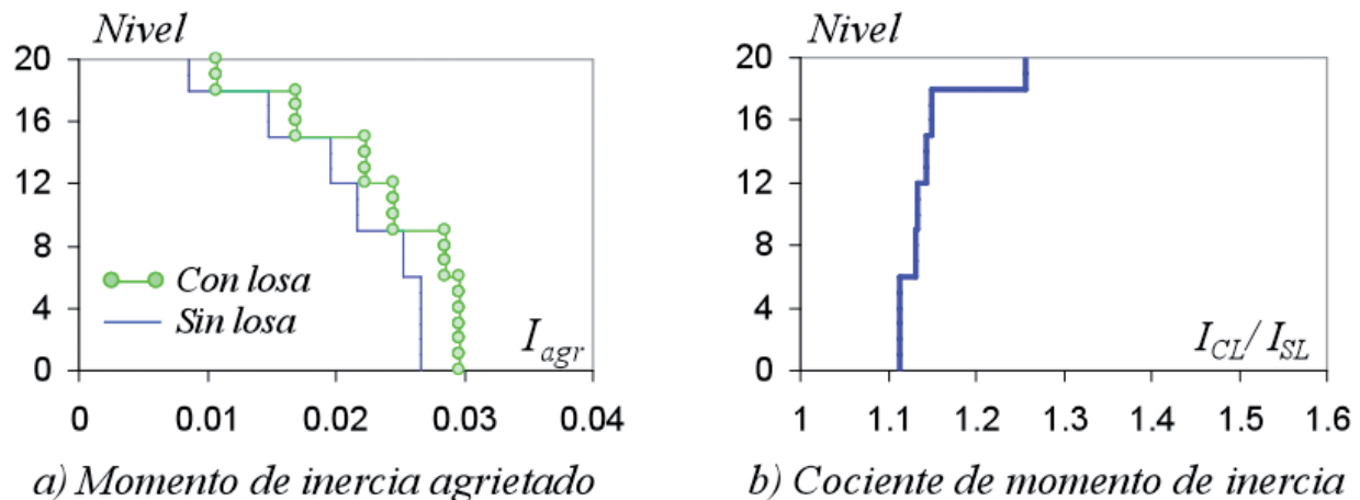
Fig. 6. Efecto de la losa en el momento de inercia agrietado de las vigas de los marcos internos del edificio de veinte pisos.
