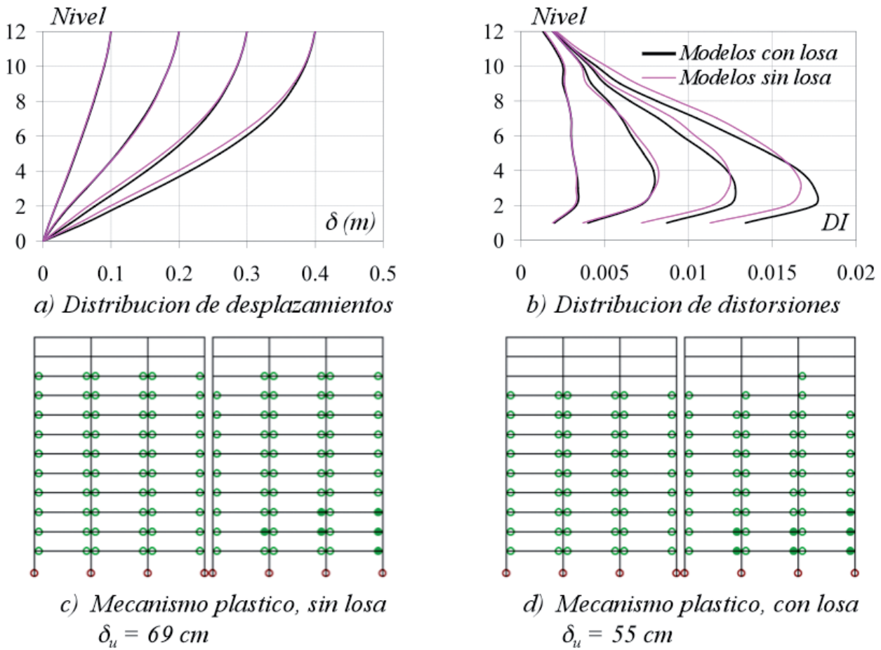
Fig. 9. Distribución de deformaciones laterales en altura y mecanismos plásticos para el edificio de doce pisos.
