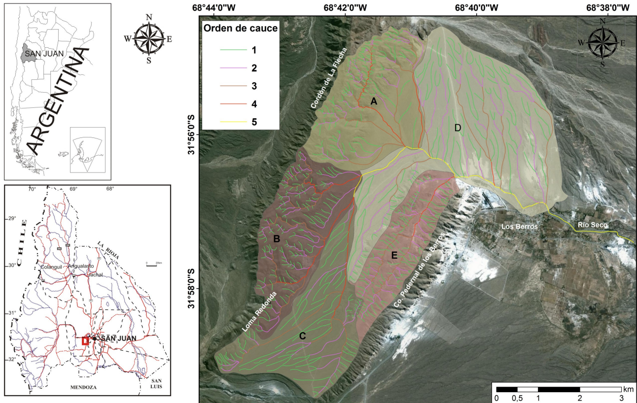
Figura 1. Ubicación del área de estudio y cuenca de 5 o orden del río Seco. La cuenca ha sido subdividida en 5 sub-cuencas, identificadas con letras mayúsculas desde la A a la E, (Esper Angillieri, 2014).
