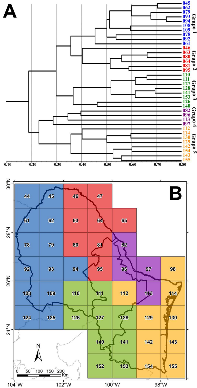
Figura 2. A) Similitudes florísticas entre los cuadros en que se dividió la región noreste de México. B) Distribución geográfica de los cinco grupos florísticos (fitocorias) identificados mediante el análisis de agrupamiento.
