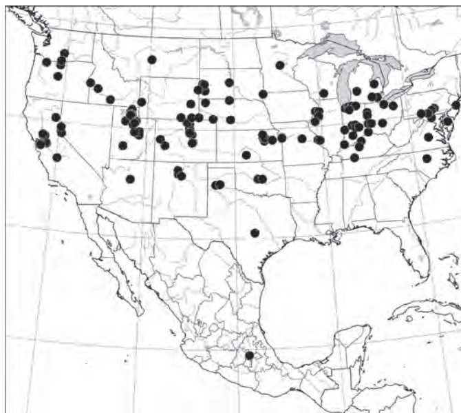
Figura 3. Mapa de localidades de colecta para Scolystus schevyrewi en los Estados Unidos y México.
