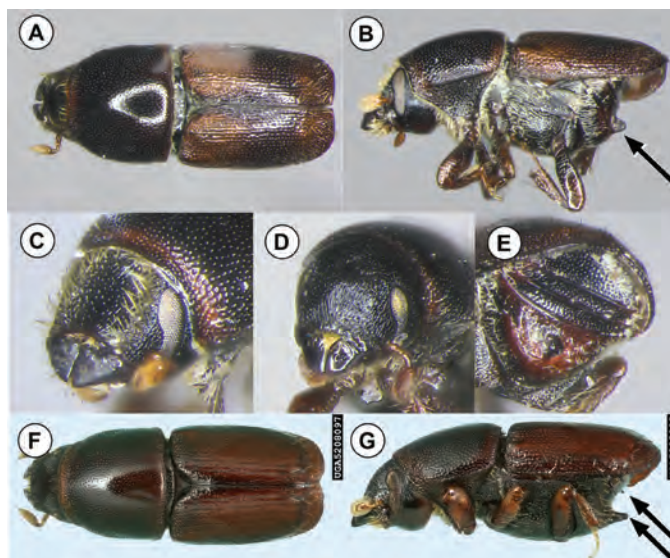
Figura 4. Comparación entre Scolystus schevyrewi y S. multistriatus . A) S. schevyrewi : vista dorsal del macho, B) S. schevyrewi : vista lateral del macho, C) S. schevyrewi : frente del macho, D) S. schevyrewi : frente de la hembra, E) S. schevyrewi : vista ventro-abdominal del macho F) S. multistriatus : vista dorsal de la hembra, G) S. multistriatus : vista lateral de la hembra. Fotos A-E Tomadas por T.H. Atkinson. Fotos F-G Tomadas por N. Wright, Florida Department of Agriculture and Consumer Services ( http://www.insectimages.org/browse/detail.cfm?imgnum=5208097 ).
