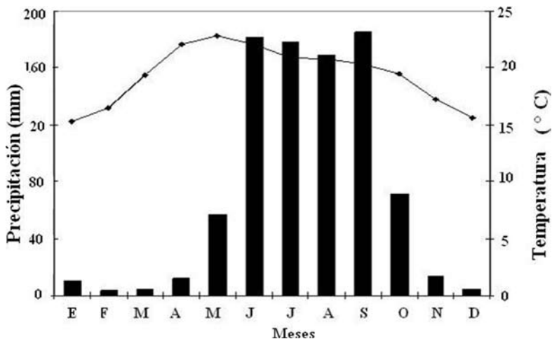
Figura 1. Climograma de la estación climatológica Yauatepec, Morelos (18° 53' 0.15" N, 99° 04' 3" O). Las barras oscuras representan la precipitación y la línea la temperatura.
