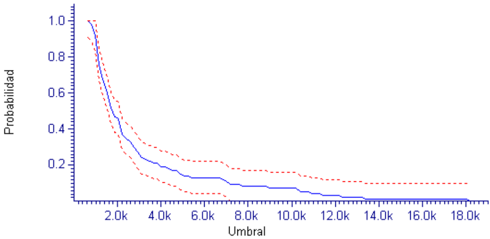
Figura 7. Disminución en la probabilidad del crecimiento poblacional de Crocodylus moreletii en la UMA Cacahuatal. Los valores del rango del umbral de la capacidad de carga ( k ) son de 1.2k y 18k, que representan una probabilidad de disminución poblacional que va de 0.9 a 0, respectivamente. La línea punteada roja denota el valor máximo y mínimo (por encima y debajo de la línea de tendencia, respectivamente) del umbral esperado de k .
