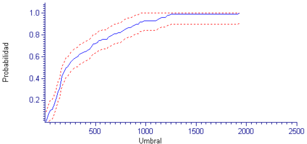
Figura 8. Aumento en el riesgo de extinción en la población de Crocodylus moreletii de la UMA Cacahuatal. El valor del umbral poblacional inicial es de ~40 cocodrilos que conllevaría a la extinción de la población. La línea punteada roja denota el valor máximo y mínimo (por encima y debajo de la línea de tendencia, respectivamente) del umbral esperado de la población.
