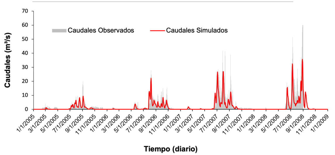
Figura 7. Eficiencias obtenidas con el modelo hidrológico TETIS en el periodo de validación. Fuente: Orozco et al. (2020).
