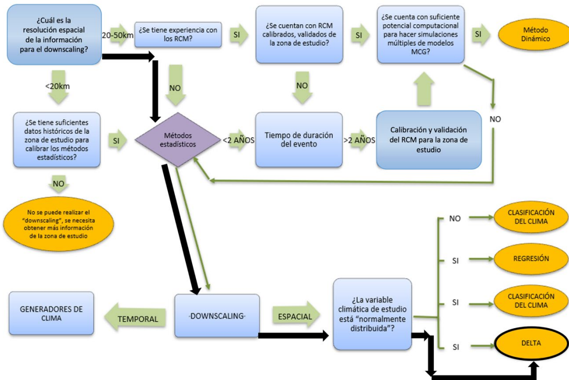
Figura 5. Diagrama de flujo usado para la selección de la metodología downscaling a emplear en la investigación. Fuente: Trzaska et al. (2014).
