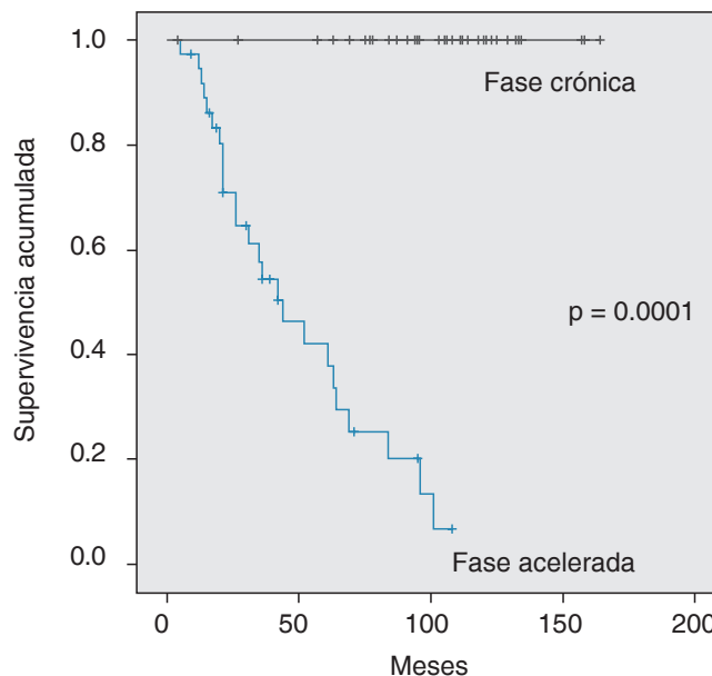
Figura 2: Supervivencia global
